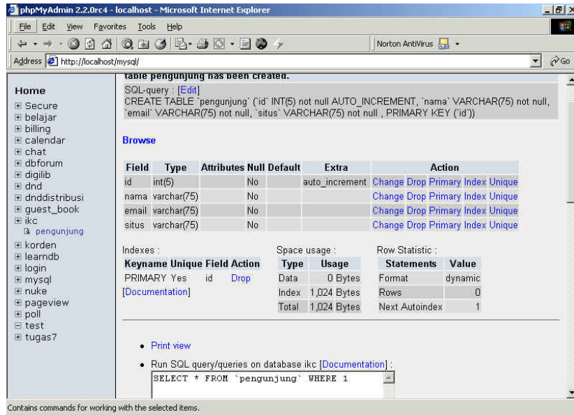
Gambar 5: Tabel pengunjung
