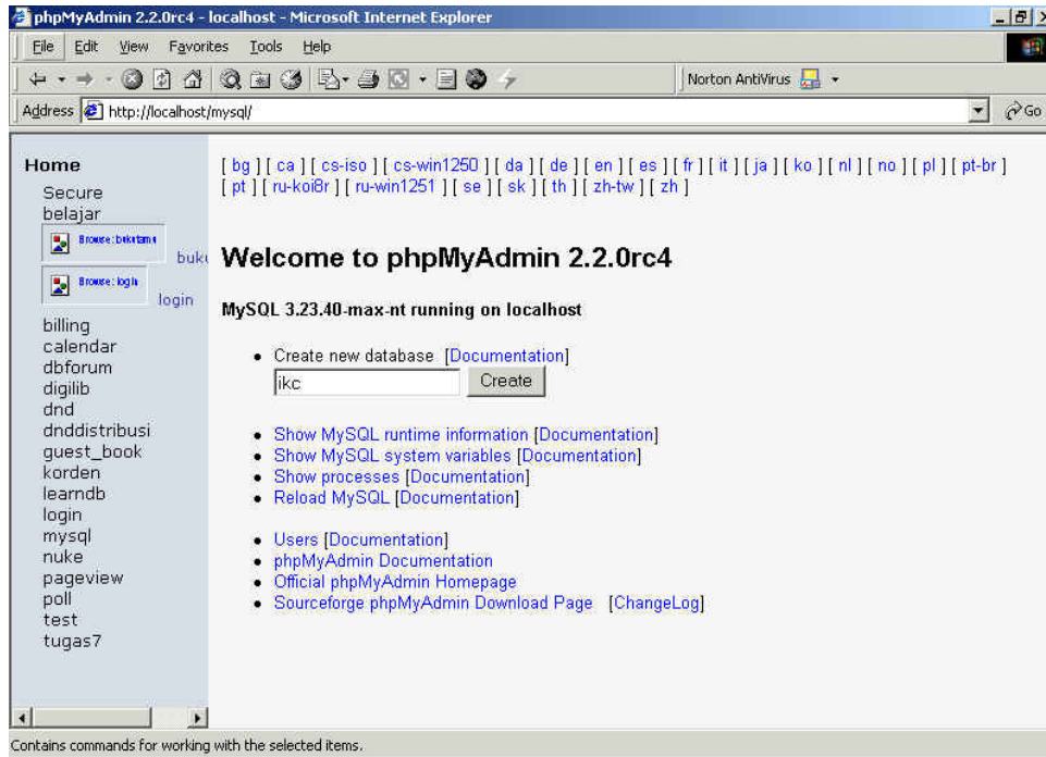
Gambar 1: Database baru
